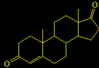
4-androstenedione
