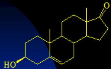
DHEA
