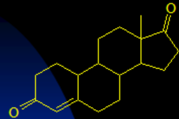
19-Nor-4-androstenedione
